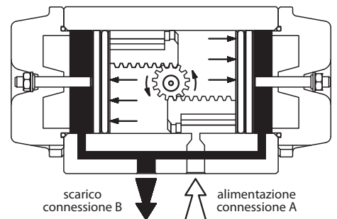
Movimento pistoni in apertura, rotazione antioraria quando alimentazione in connessione A
